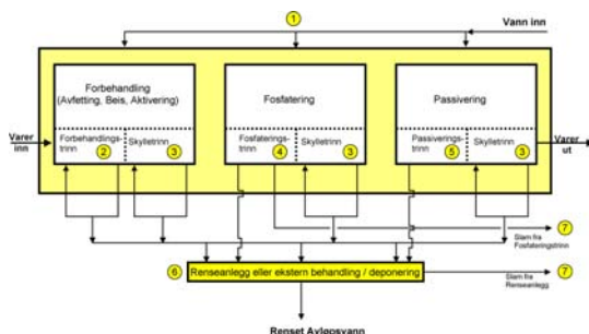
Bildet viser eksempel på forbehandlings anlegg for pulverlakk
